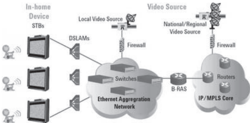
ตัวอย่าง Network Architecture ของโทรทัศน์ไอพี (IPTV)
