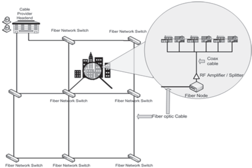
ตัวอย่าง Network Architecture ของโทรทัศน์ทางสาย (Cable TV)
