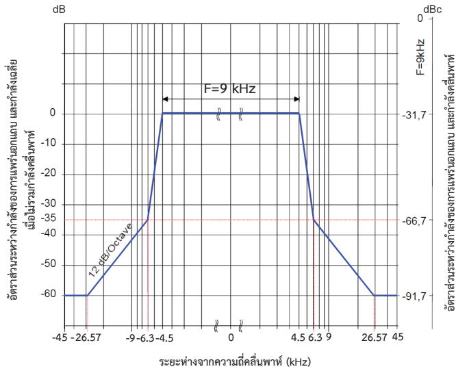
รูปที่ 1 ขอบเขตการแผ่รังสี
