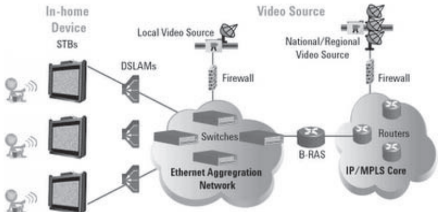
ตัวอย่าง Network Configuration ของโทรทัศน์ไอพี (IPTV)
