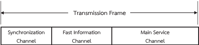
รูปที่ 2 โครงสร้างเฟรมส่งสัญญาณ
