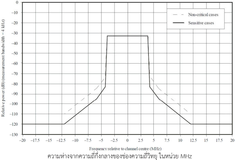
รูปที่ 2 กรอบของการแพร่กระจายคลื่น (Spectrum Mask)
