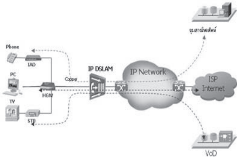
ตัวอย่าง Network Architecture ของโทรทัศน์ไอพี (IPTV)
