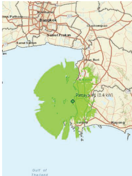
รูปที่ 5 พื้นที่การกระจายเสียงอ้างอิงของสถานีวิทยุคมนาคม Pattaya - N1
