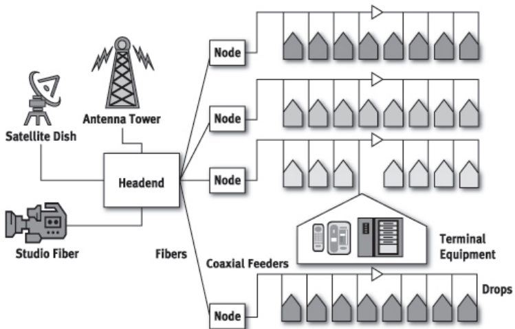
ตัวอย่าง Network Configuration ของโทรทัศน์ทางสาย (Cable TV)
