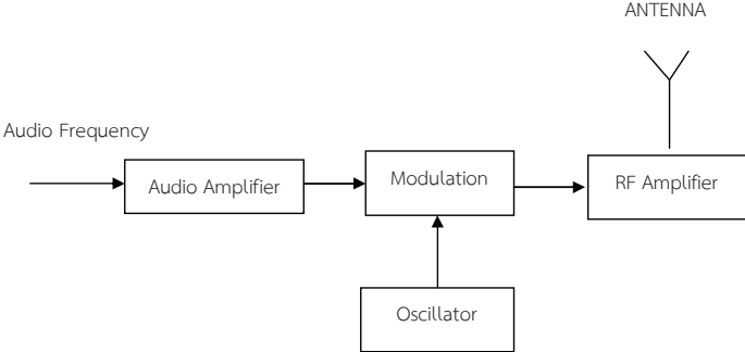
ตัวอย่าง Network Configuration ของวิทยุกระจายเสียงในระบบแอนะล็อก
