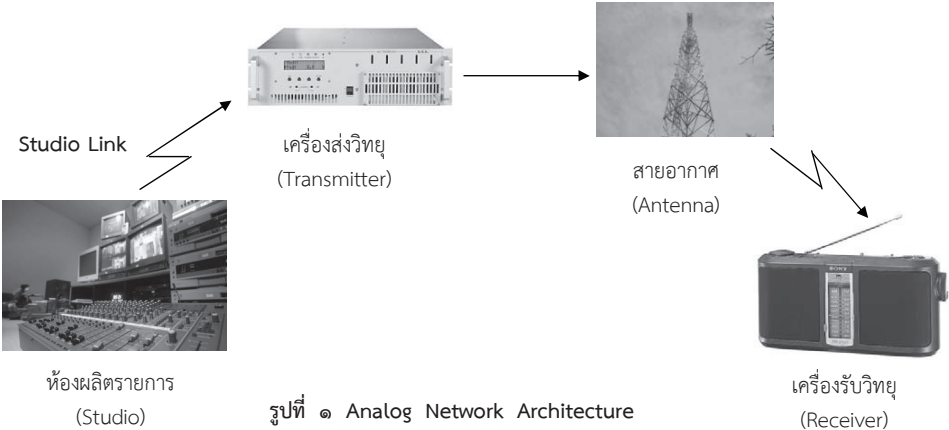
ตัวอย่าง Network Configuration ของวิทยุกระจายเสียงในระบบแอนะล็อก
