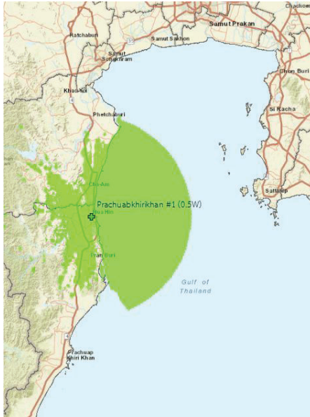
รูปที่ 12 พื้นที่การกระจายเสียงอ้างอิงของสถานีวิทยุคมนาคม Hua Hin - N1
